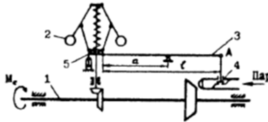
Рис. 1.1. Система автоматического регулирования угловой скорости паровой турбины
