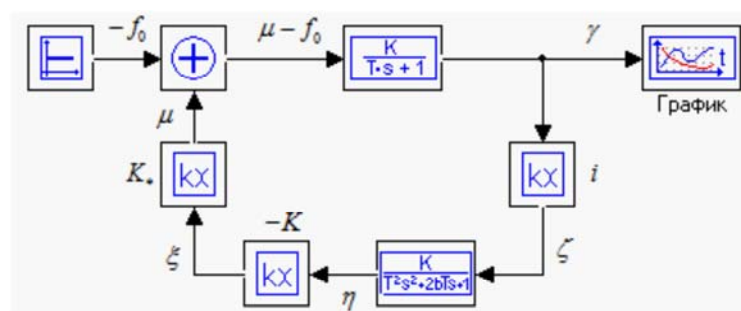
Рис. 1.5. Структурная схема
